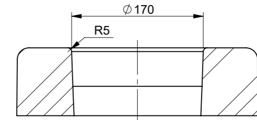
SECTION A-A SCALE 1 : 5
