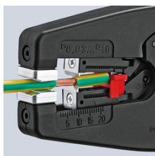
Trådavbitare till 10 mm 2 flertrådig
