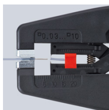
Exakt avisolering från 0,03 till 10 mm 2 utan efterjustering
