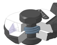
Inliggande öppningsfjäder
