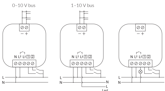
Koppling för 0–10 V bus (utan brytning av matning till last)
