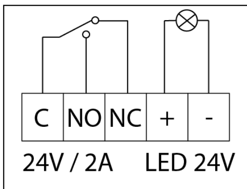
Inkopplingsanvisning
