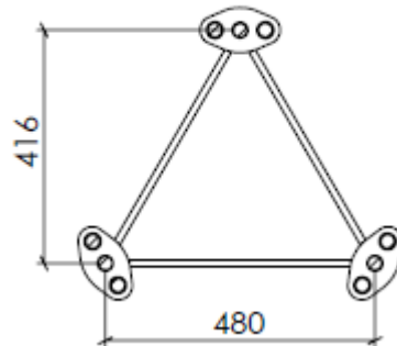
SECTION B-B SCALE 1 : 12
