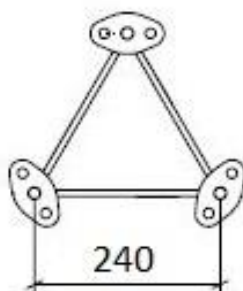
SNITTVY B-B SKALA 1 : 10
