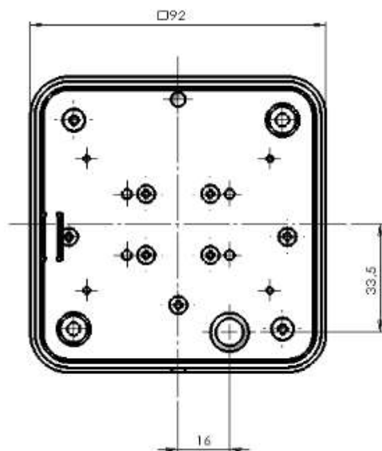
Måttritning styrenhet för kabelgenomföring från baksidan
