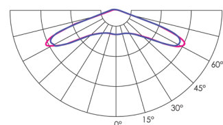
Symmetrisk 21 W LED 2685lm 4000K RAL9007 Artikelnr 7750128
