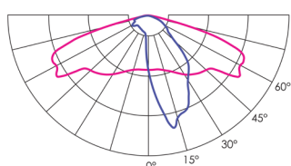
Asymmetrisk 13 W LED 1971lm 4000K RAL9007 Artikelnr 7750130
