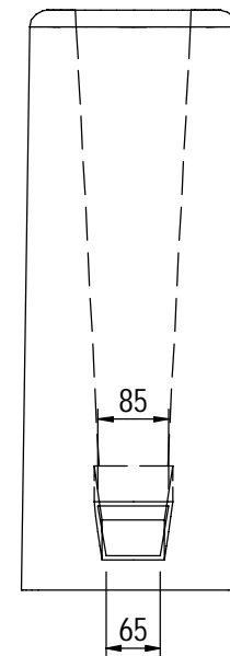
B-B 1 : 10
