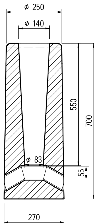
A-A 1 : 10
