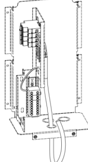
Elddragning laddbox
