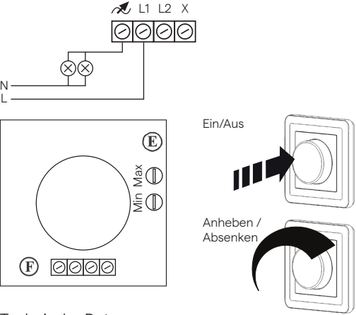
Anschlussplan
