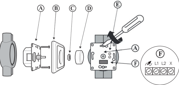
Anschlussplan
