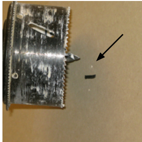
Använd 74mm multifräs och gör ett spår i skivväggen över den ena markeringen från piggarna.
