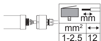
DALI
