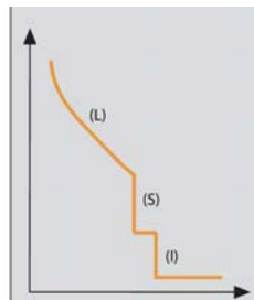
LSI-skydd
