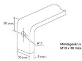
Mått anslutningsskena
