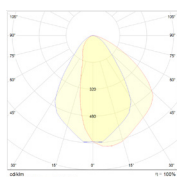
36W Asymmetrisk
