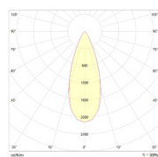
20W Symmetrisk
