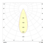
36W Symmetrisk
